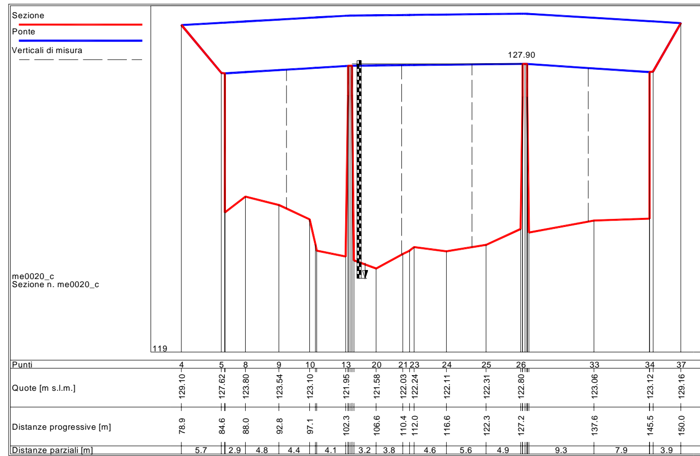
Sezione idrometrica me0020_c
