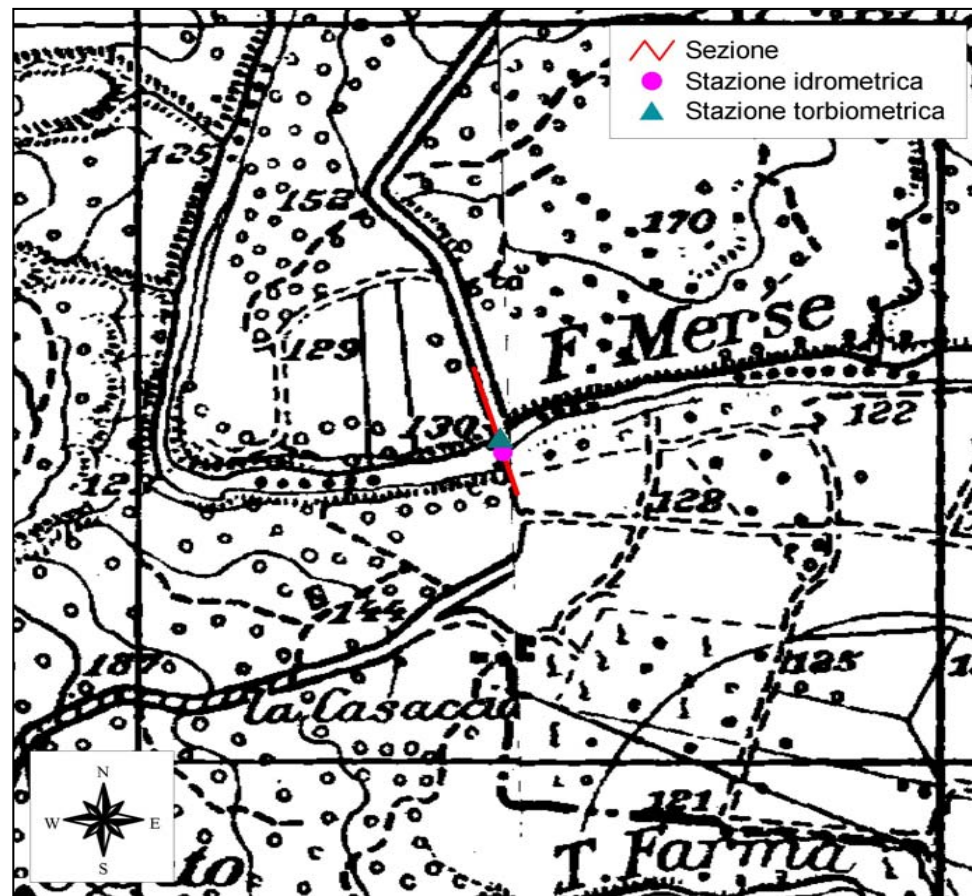
Planimetria in scala 1:10000 della sezione a Ponte a Montepescini.
