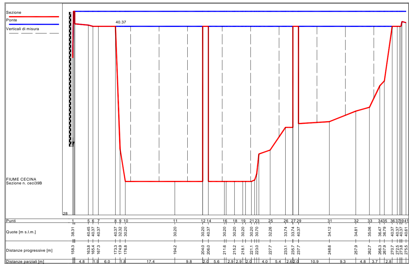
Sezione idrometrica ceci39b
