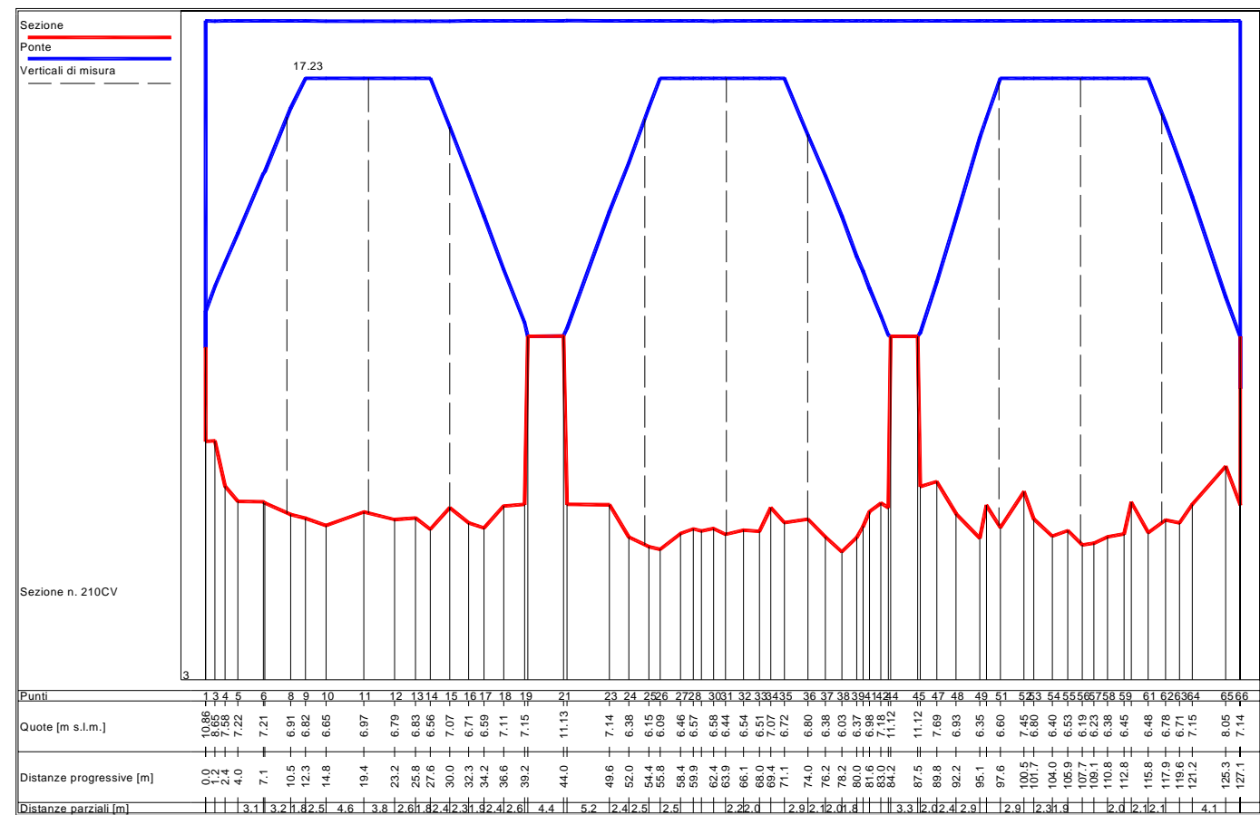
Sezione idrometrica 210CV
