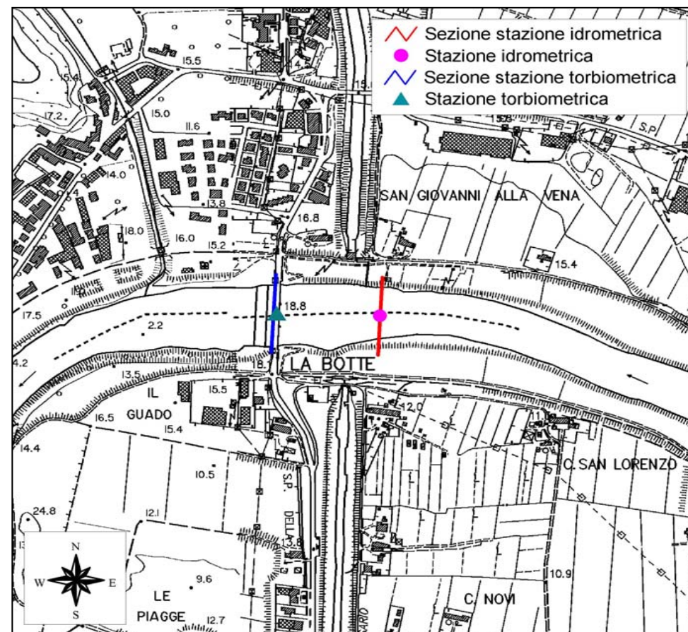
Planimetria in scala 1:10000 della sezione a San Giovanni alla Vena.
