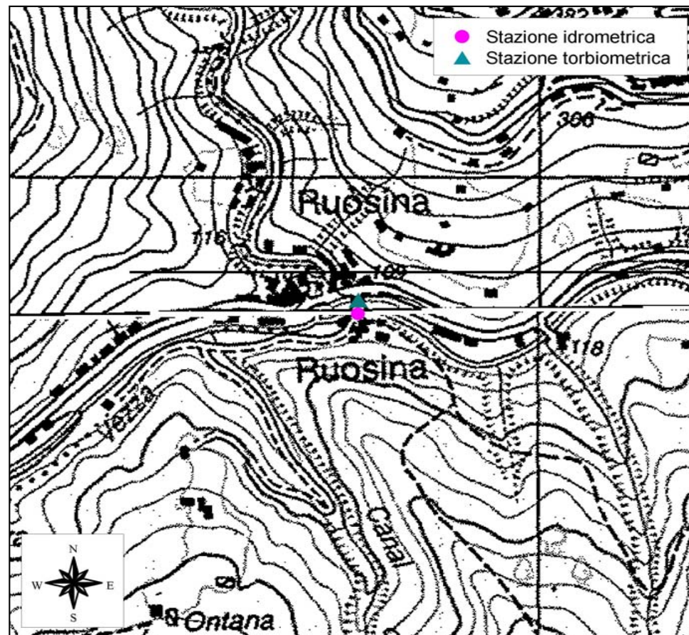
Planimetria in scala 1:10000 della sezione a Ruosina.
