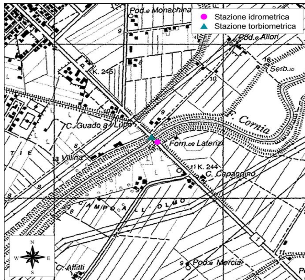
Planimetria in scala 1:xxxxxx della sezione a Ponte ex SS n°1.
