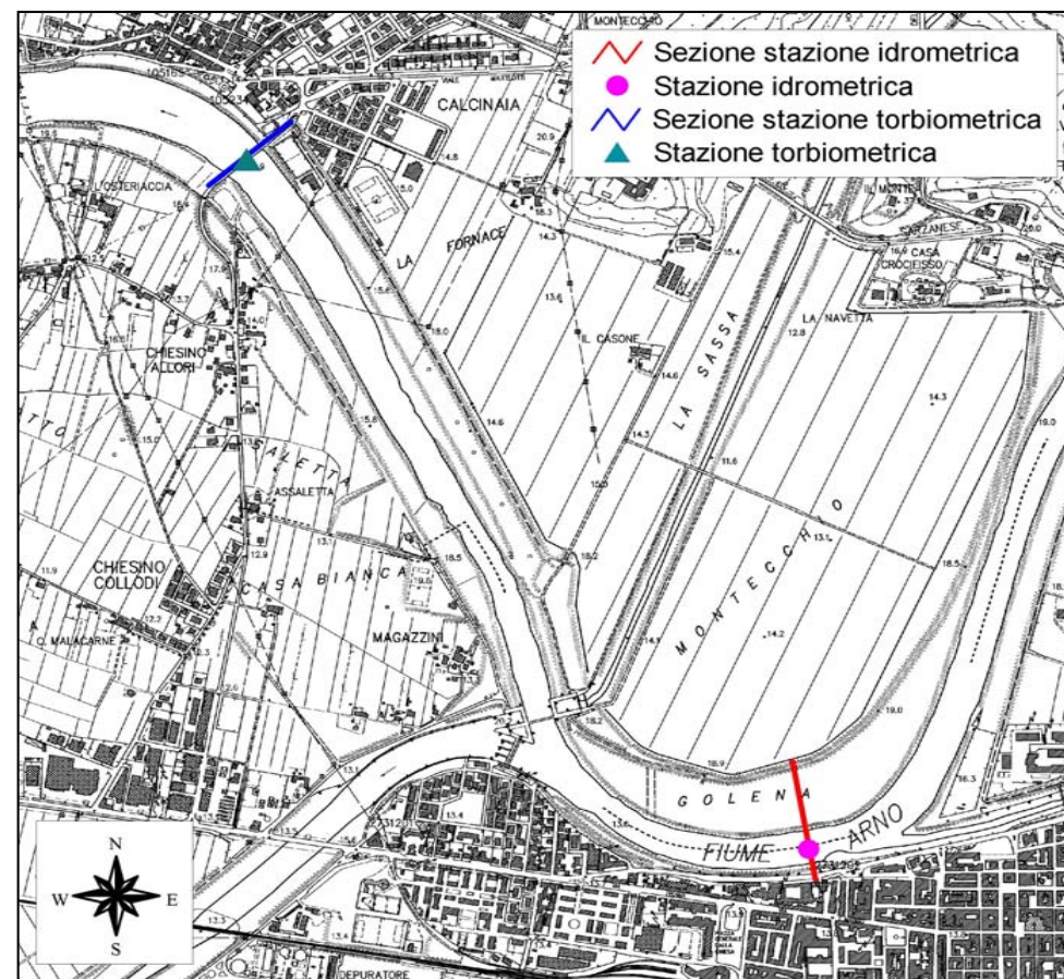
Planimetria in scala 1:20000 della sezione a Leoncini.
